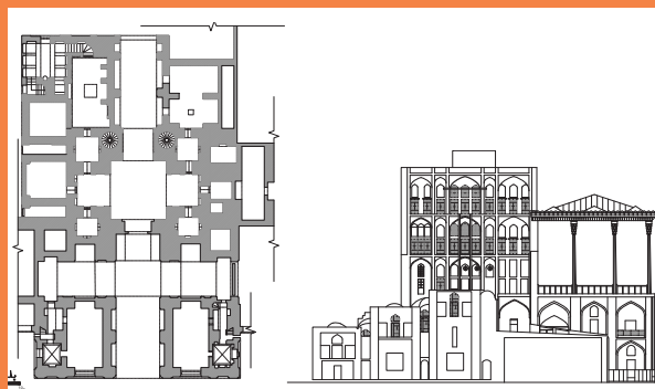
نقشه کاخ عالی قاپو (معروف به قصر دولت خانه) موقعیت: ضلع غربی میدان نقش جهان اصفهان، مشخصات: ۴۸ متر ارتفاع در ۶ طبقه سال ساخت: بین سالهای ۹۷۳ تا ۹۷۷ خورشیدی (دوره شاه عباس اول)، قدمت: ۴۲۰ سال معمار بنا: استاد علی اکبر اصفهانی، مینیاتورست بنا: رضا عباسی
