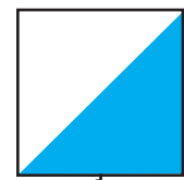
شکل ۱۵: نصفش را در نظر بگیر
