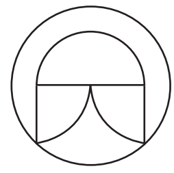
شکل ۱۴ب: ترکیب دوباره ربع دایره‌های نیم دایره
