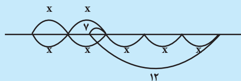
شکل ۱۷: نمایش 2x - 7 = 5x - 12
