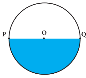
ب شکل ۱۸: دو حالت اکستريم (و متقارن)
