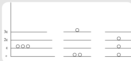
شکل ۱ سه راه توزیع مختلف برای یک سامانه سه ذره‌ای با انرژی E=3E آنتروپی سامانه، با چنین انرژی برابر با S = k \ln 3 است.
