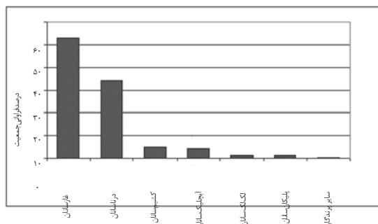
نمودار ۲. فراوانی جمعیت گروه‌های عمده پرنده‌ها در تالاب چغاخور
