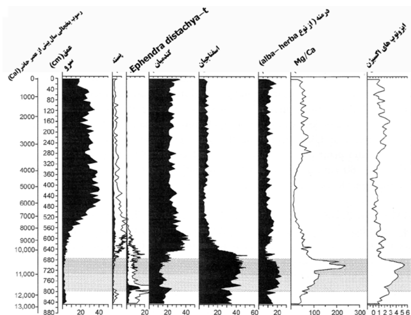
شکل ۵. نمودار گرده‌ای مرداب چاب، برگرفته از نیکلوسکی و وان‌زنیست (۱۹۷۰). استخراج از پایگاه اطلاعات گرده‌شناسی اروپا. سن ۱۱/۳۵۳ هزار سال پیش از عصر حاضر کربن پرتوزای تنظیم شده، به دلیل تأثیر آب سخت، قدیمی‌تر از آن به نظر می‌رسد. منطقه‌ی سایه روشن نشان‌دهنده‌ی دریای جوان‌تر است.
