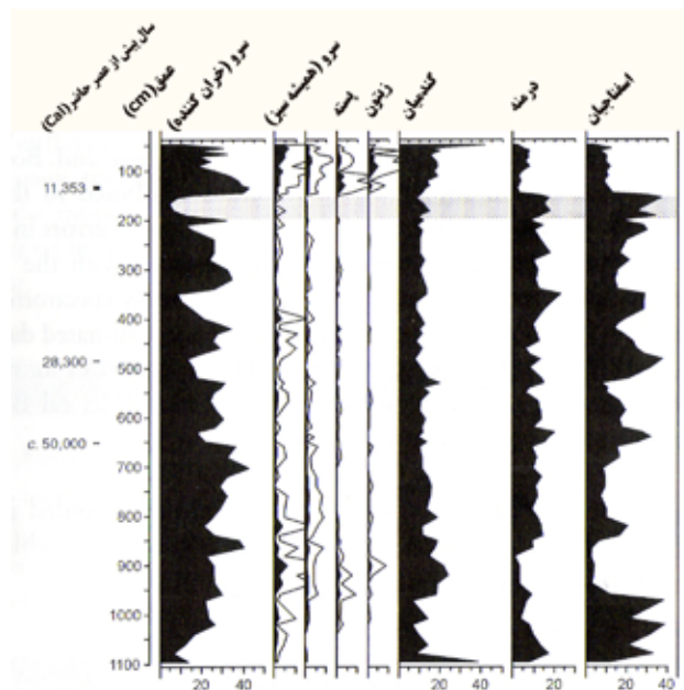
شکل ۷. نمودار گردهای دریاچه‌ی هوله. باز ترسیم از باروچ و بوتما (۱۹۹۹) با سن‌های کربن پرتوزای تصحیح شده به وسیله‌ی کاپر و همکارانش (۲۰۰۱) و نیز سن‌های تنظیم شده. منطقه‌ی سایه‌روشن نشانگر درایای جوان‌تر است.
