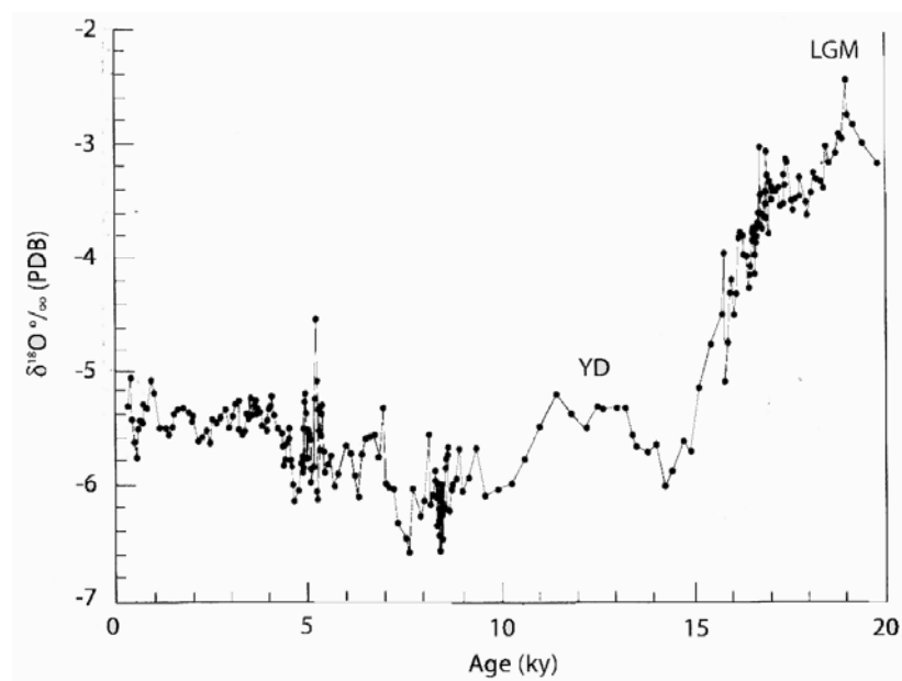
شکل ۸. چینه‌شناسی \delta^{18}\text{O} برای غار نهشته‌هایی از غار سورک. سن‌ها بر پایه‌ی تحلیل‌های اورانیوم و تورיום تعیین شده‌اند. بنابراین سال‌های تقویمی فرضی LGM: بیشینه‌ی یخچالی پسین YD: درایای جوان‌تر هستند.
