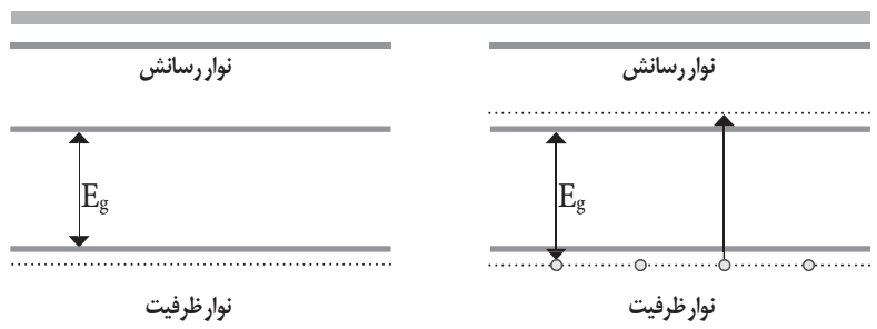
شکل ۱. مواد نیم‌رسانا در دمای صفر مطلق و دمای بالاتر
