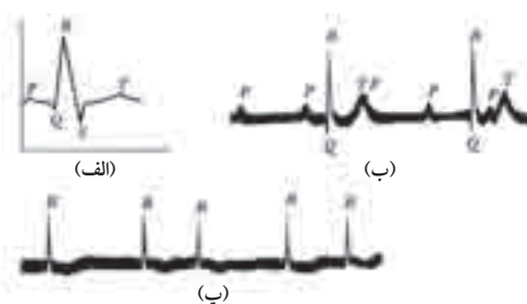
شکل ۴. EKGهای غیرعادی
