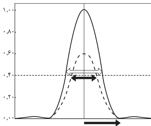
شکل ۴. نمودار شدت نور برحسب شعاع برای ستارگان با روشنایی‌های مختلف. شعاع قرص ابری برای هر دو ستاره یکسان است، اما به علت آستانه آشکارسازی چشم (خط نقطه‌شین)، بیشینه مرکزی مری (بالاترین پیکان) بزرگ‌تر از ستاره کم‌نورتر (دومین پیکان) است. هر دو ستاره گرد و دارای اندازه معین به نظر می‌رسند، اما ستاره روشن‌تر بزرگ‌تر به نظر می‌آید. هر دو ستاره به واسطه بزرگ‌نمایی بزرگ شده‌اند.
