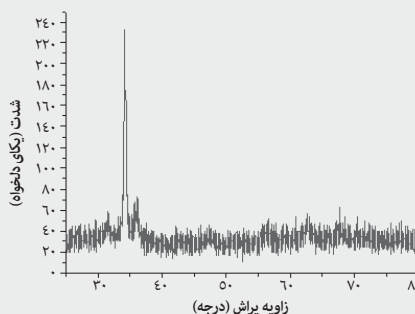
شکل ۲: طرح پراش پرتو X برای لایه های بلورین اکسید روی
