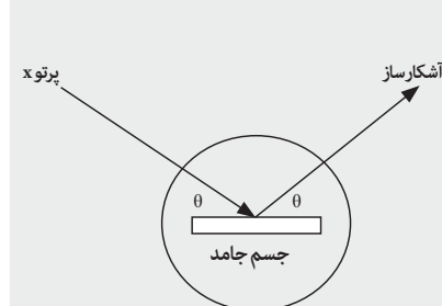
شکل ۱: پراش پرتو X به وسیله یک جسم جامد
