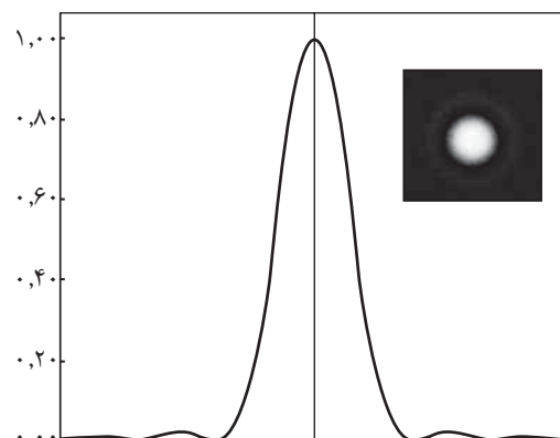
شکل ۳. نمودار شدت نور برحسب شعاع طرح پراش یک روزنه دایره‌ای (تصویر پیوست)، شعاع قرص ابری را نشان می‌دهد که در آن شدت نور برای اولین بار به صفر فرو می‌افتد. از لحاظ نظری باید شدت نور فقط در شعاع ابری صفر شود، اما در این حالت اولین منطقه تاریک پنهان قابل ملاحظه‌ای دارد، یعنی اندازه بیشینه مرکزی مرئی کمتر از شعاع قرص ابری است.
