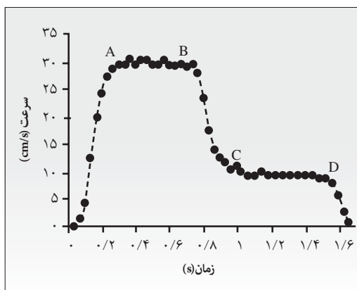
تصویر ۴: مؤلفه عمودی سرعت گلوله فولادی بر حسب زمان
