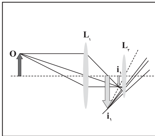
شکل ۱. در یک تلسکوپ، عدسی L_1 (شیئی) از شی O تصویر حقیقی i_1 ، سپس عدسی L_2 (چشمی) را بزرگ کرده و یک تصویر بزرگ مجازی در i_2 تشکیل می‌دهد.
