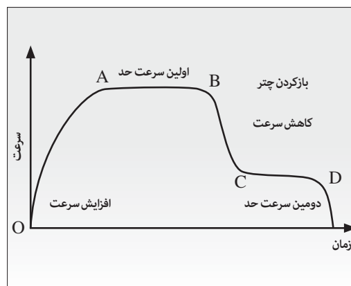
تصویر ۱: مؤلفه عمودی سرعت چتر باز در حال سقوط در هوا بر حسب تابعی زمان
