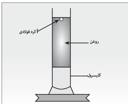
تصویر ۲: چیدمان آزمایش
